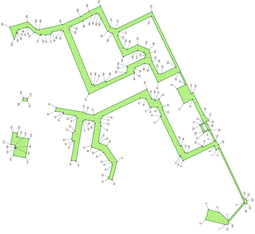
5.50. Чертеж границ публичного сервитута №11000
